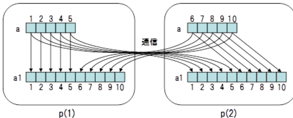
図 6: gmove の概念
